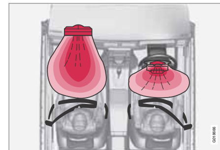
Sistema de airbags visto desde arriba, vehículo con volante a la derecha.
